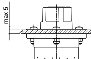
Montage interne
