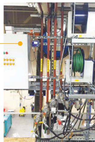
Flexible sur enrouleur avec compteur ICM intégré pour distribution de fluide
